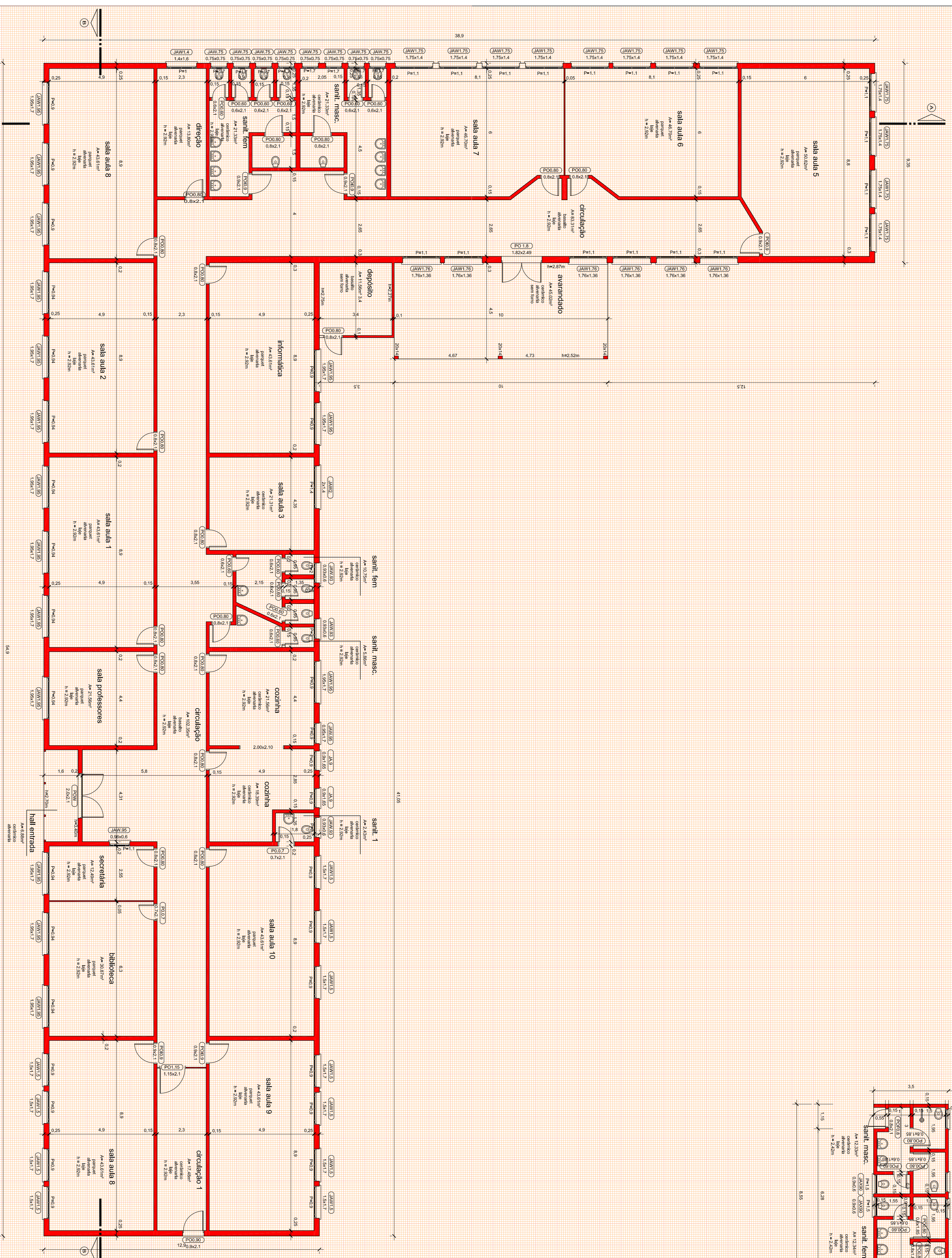
PLANTA BAIXA 1:100
