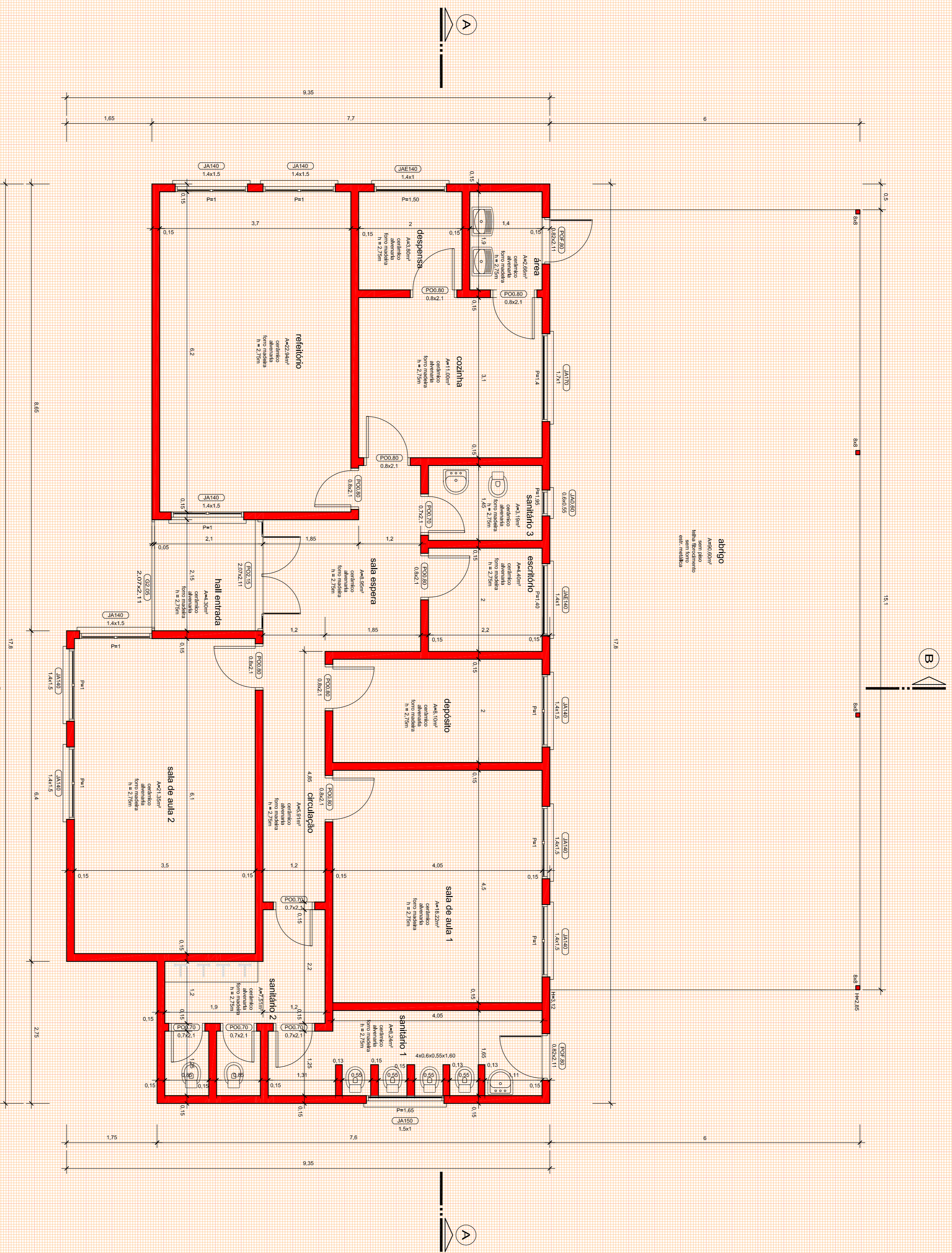
PLANTA BAIXA 1/50
