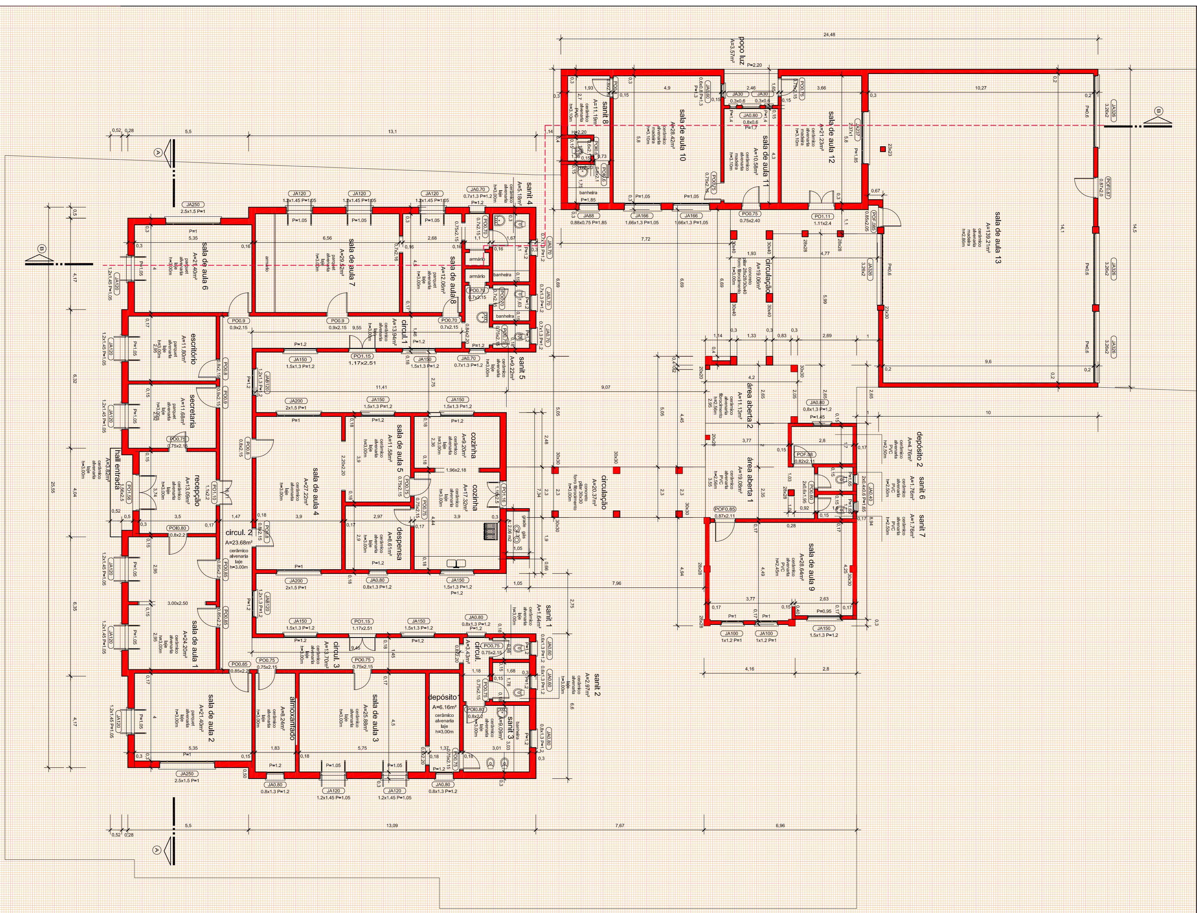
PLANTA BAIXA 1/100
