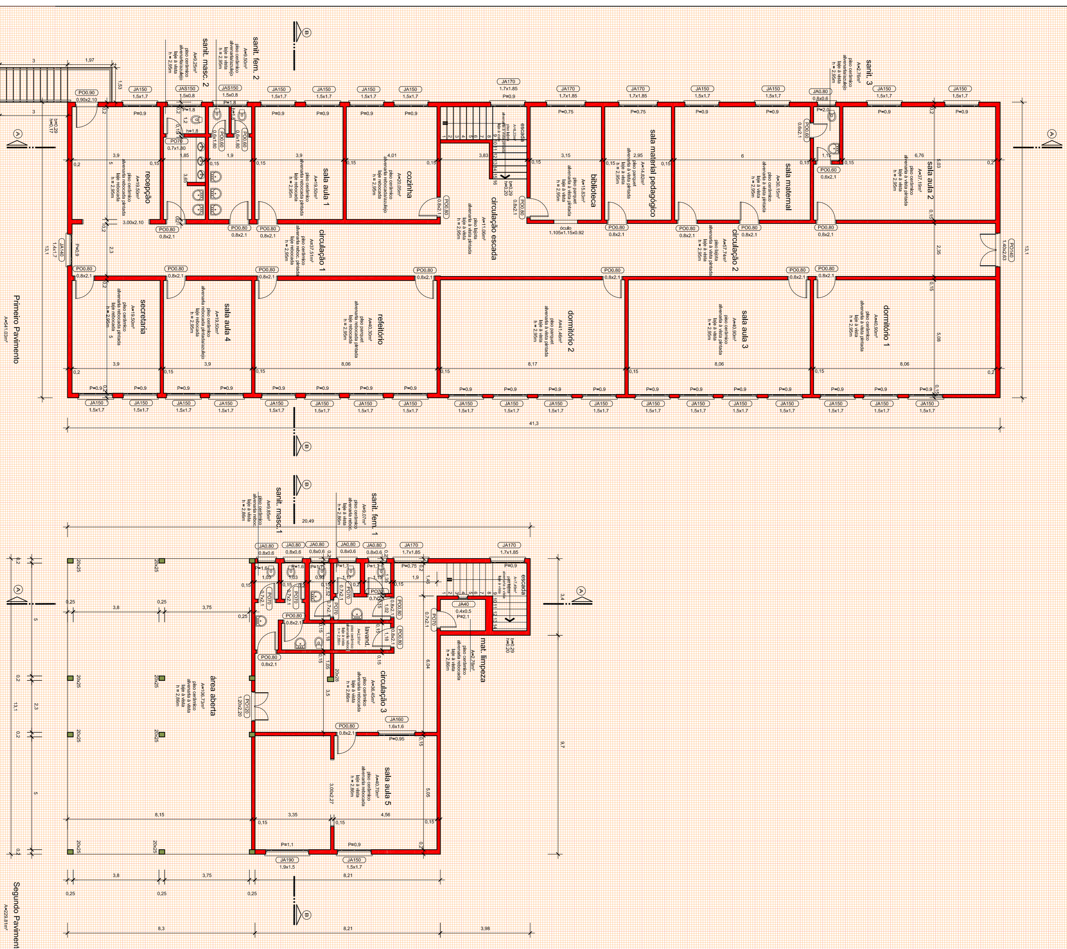
PLANTA BAIXA 1/100
