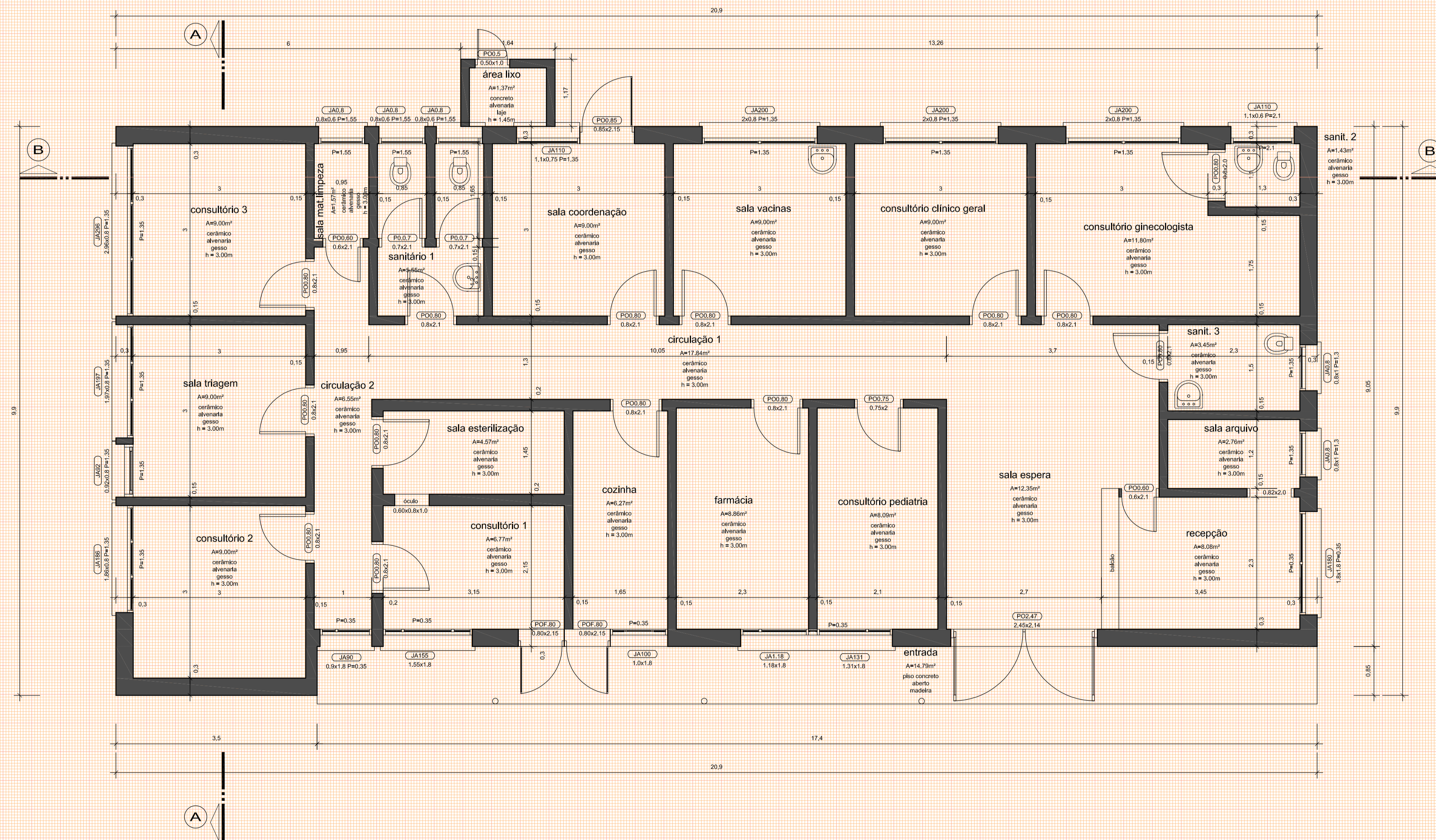
PLANTA BAIXA 1 / 50
