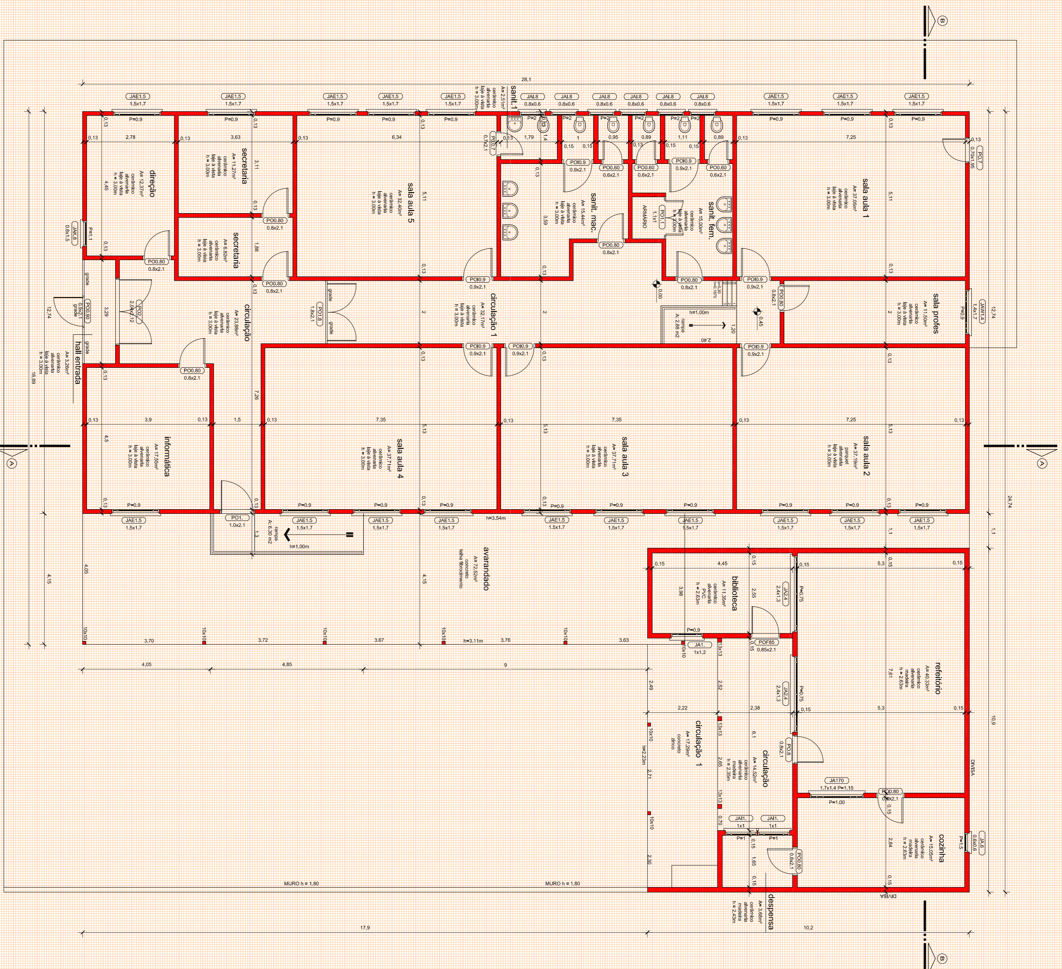
PLANTA BAIXA 1/75
