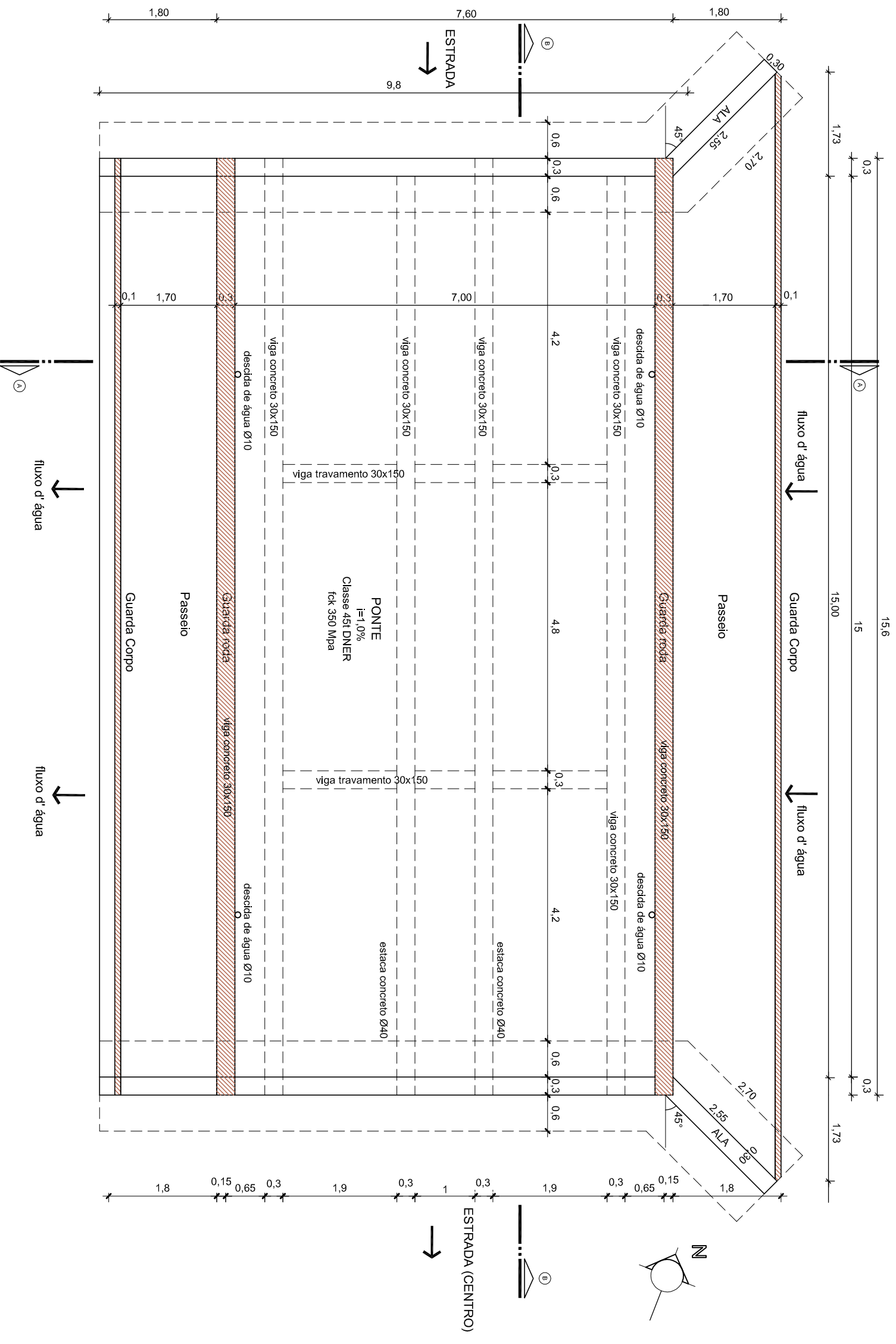
PLANTA BAIXA esc. 1/75
