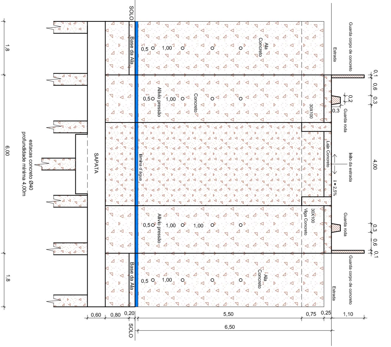
CORTE A A esc. 1/175
