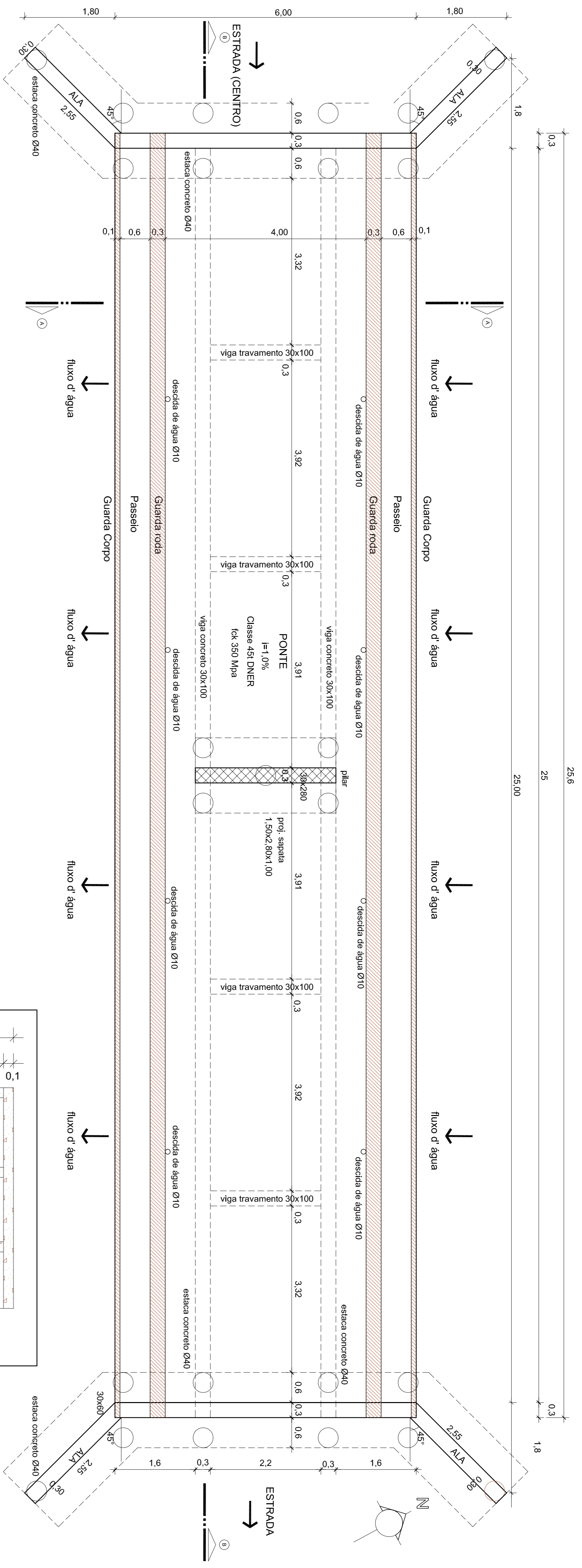
PLANTA BAIXA esc. 1/100
