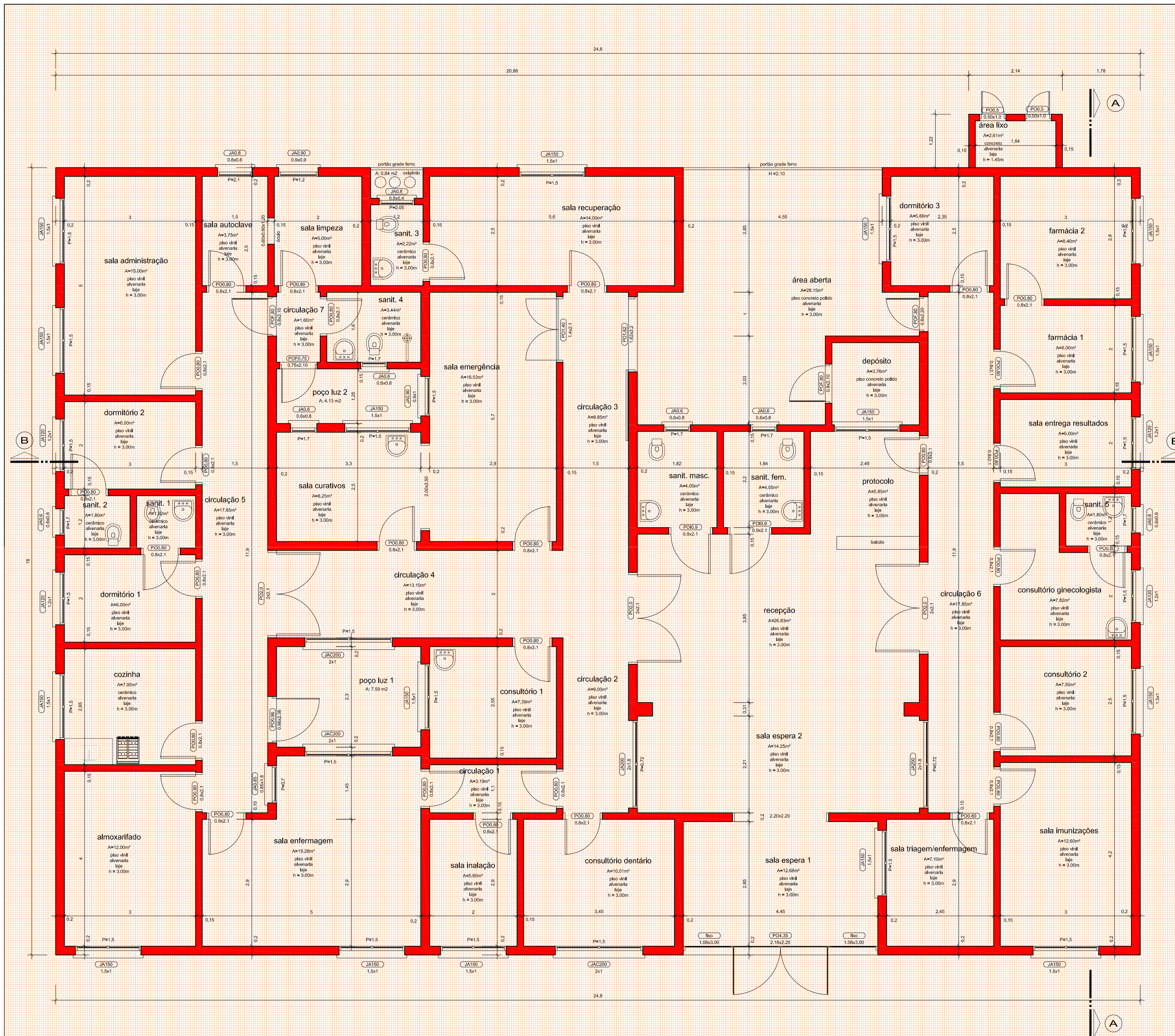
PLANTA BAIXA 1/50
