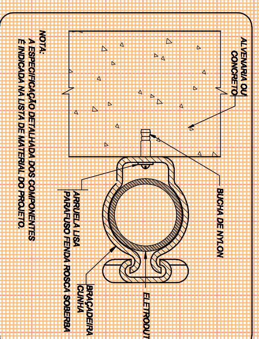
FIXAÇÃO ELETROTUBO
