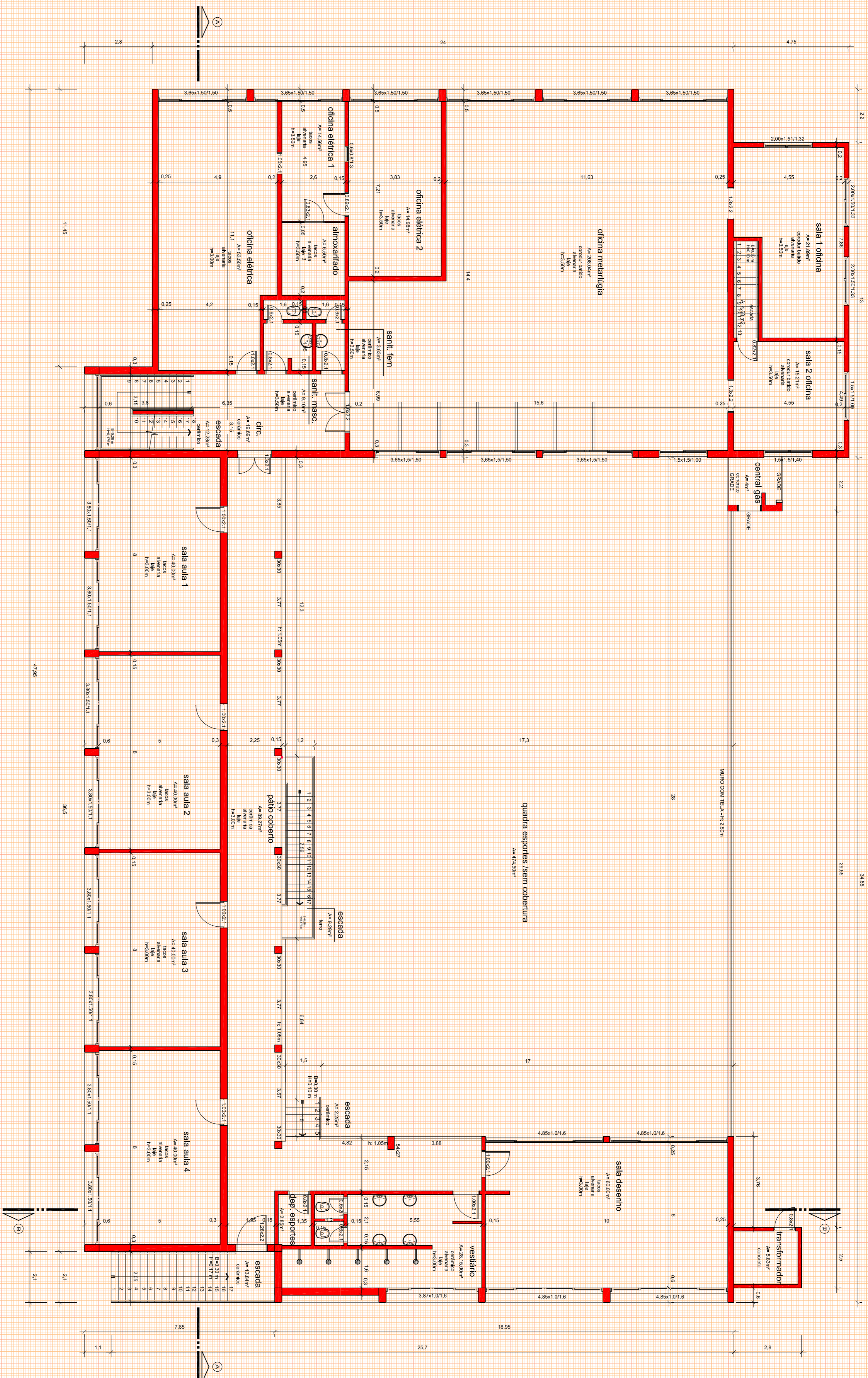
PLANTA BAIXA 2º PAVIMENTO 1 / 100
