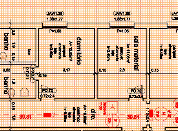
DETALHE INSTALAÇÃO SINALIZAÇÃO DE SAÍDA 1/40
